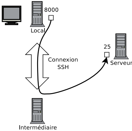
Figure 9-2 Déport d'un port local par SSH
