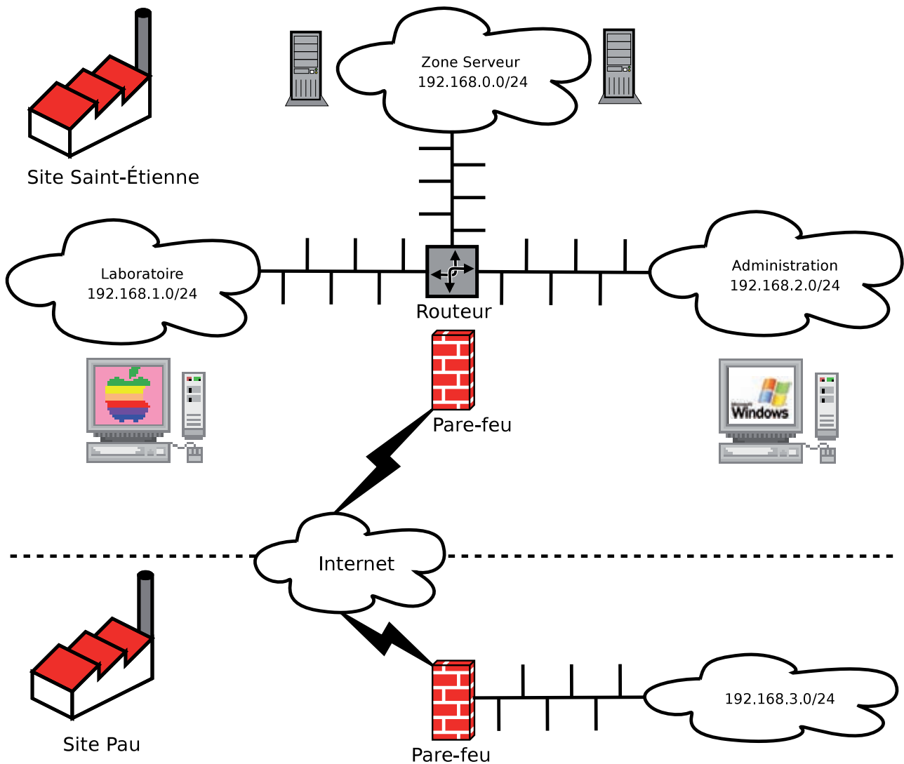
Figure 2-1 Aperçu global du réseau de Falcot SA
