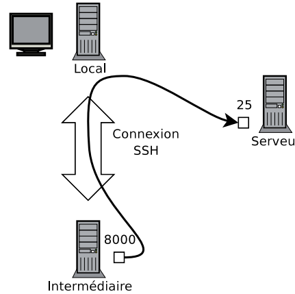
Figure 9-3 Déport d'un port distant par SSH
